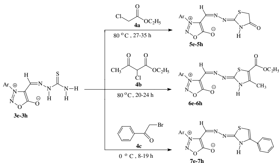
Scheme 3. 3e : Ar=C 6 H 5 ; 3f : Ar= p -CH 3 C 6 H 4 ; 3g : Ar= p -CH 3 OC 6 H 4 ; 3h : Ar= p -C 2 H 5 OC 6 H 4 .
