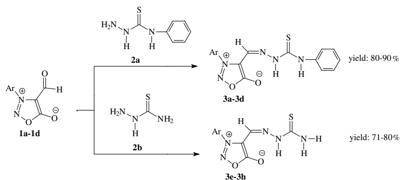
Scheme 1. 1a : Ar=C 6 H 5 ; 1b : Ar=p-CH 3 C 6 H 4 ; 1c : Ar=p-CH 3 OC 6 H 4 ; 1d : Ar=p-C 2 H 5 OC 6 H 4 .
