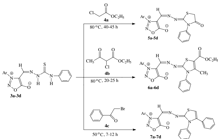
Scheme 2. 3a : Ar=C 6 H 5 ; 3b : Ar=p-CH 3 C 6 H 4 ; 3c : Ar=p-CH 3 OC 6 H 4 ; 3d : Ar=p-C 2 H 5 OC 6 H 4 .
